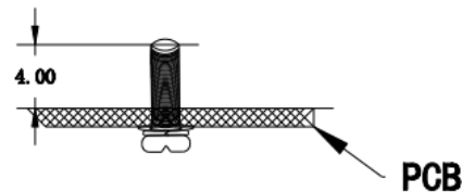
标准型 60.4*39*12.7mm
