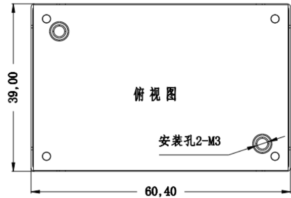
标准型 60.4*39*12.7mm
